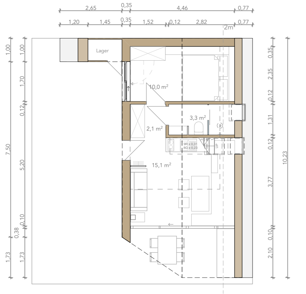
Konzept 1 EG 1:100
