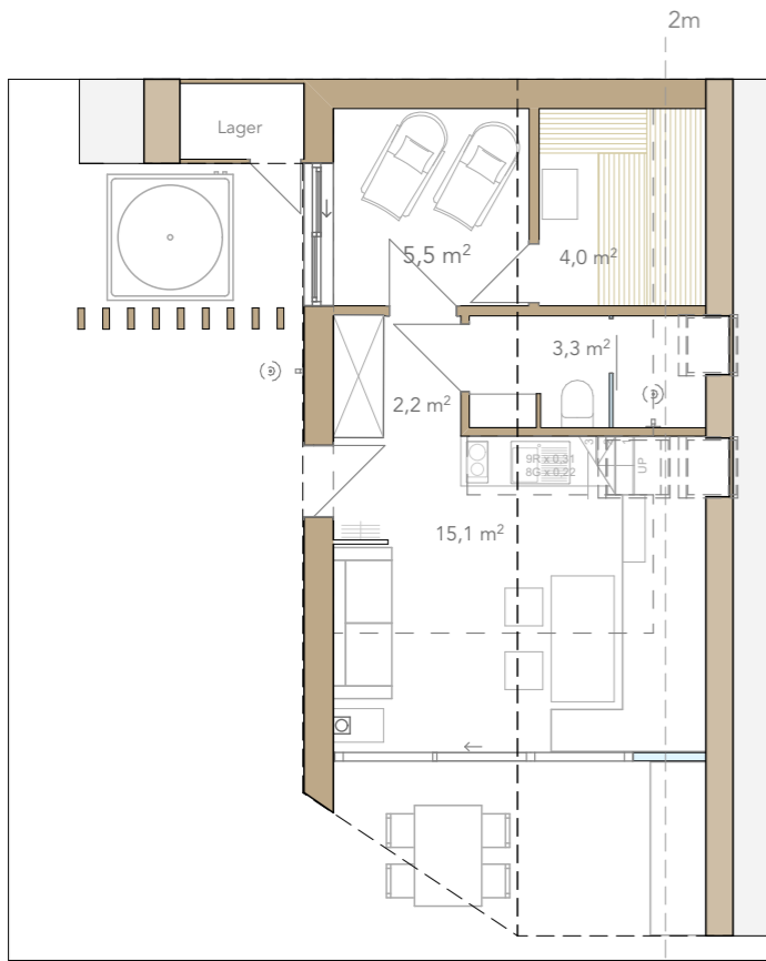
Konzept 2 EG 1:100
