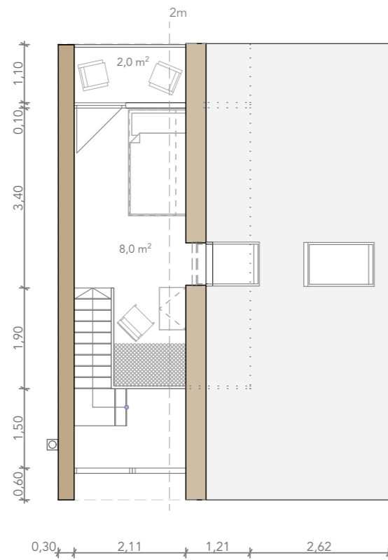
Konzept 3A Obergeschoss 1:100
