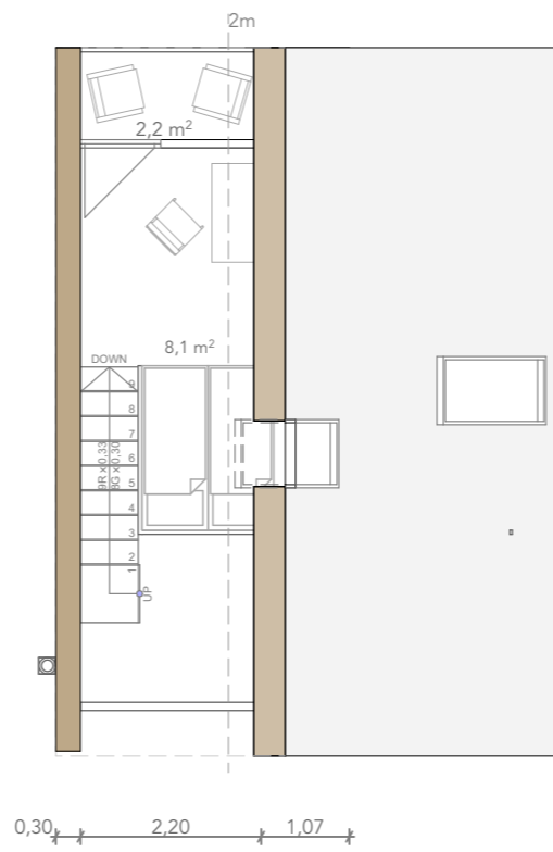
Konzept 3B 1:100
