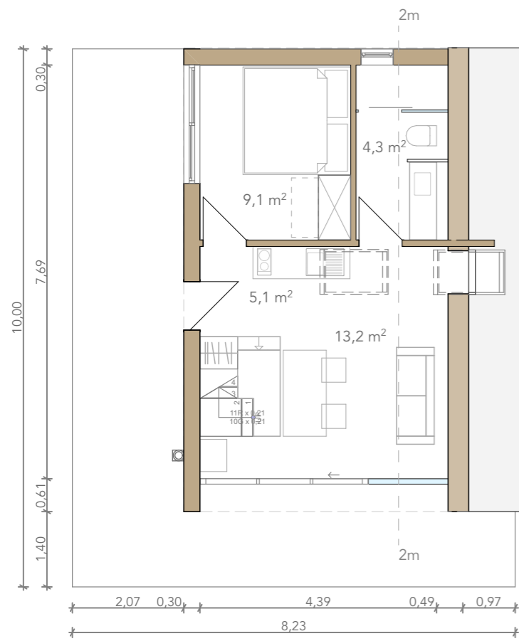
Konzept 3 Erdgeschoss 1:100
