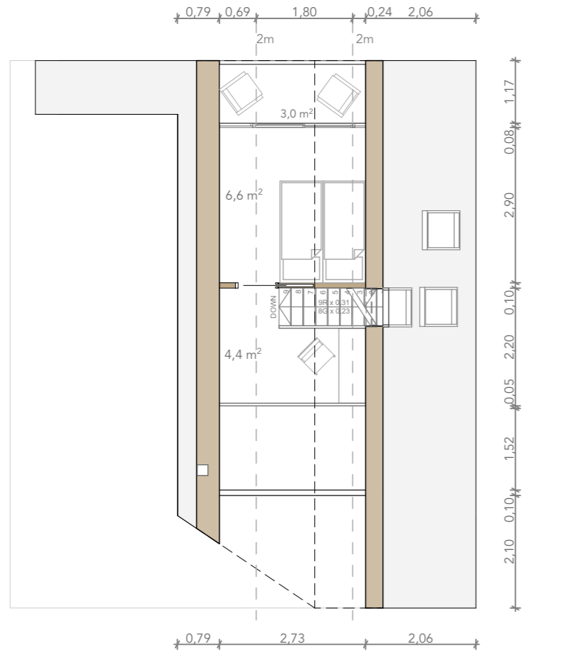
Konzept 1 OG 1:100
